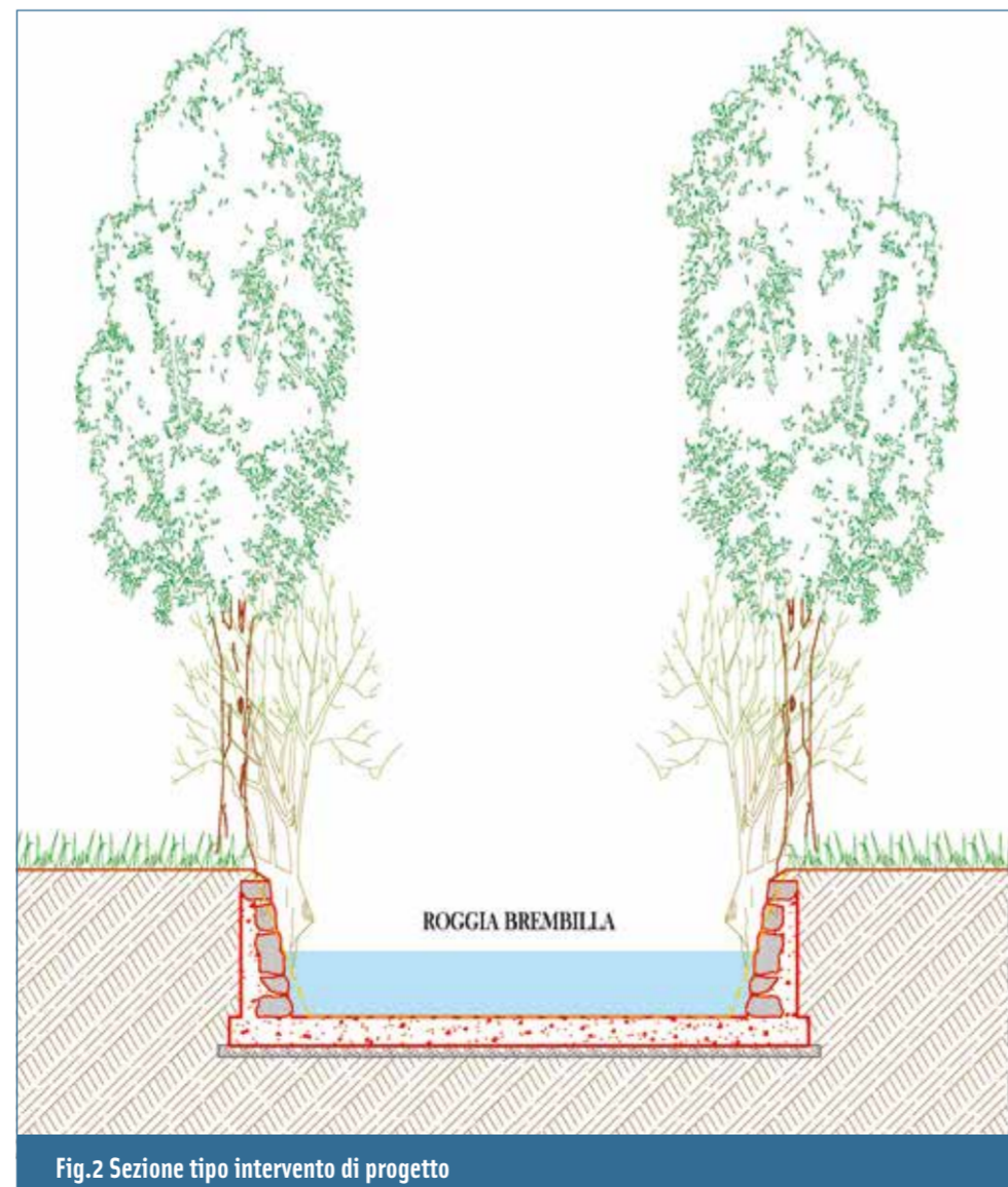
Fig.2 Sezione tipo intervento di progetto
